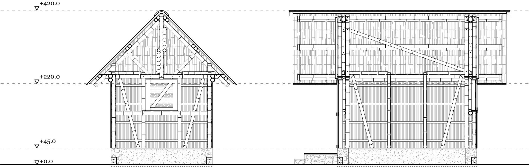
SECTION a-a'
