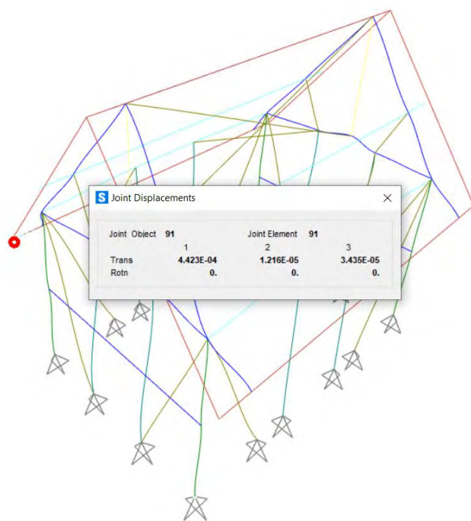
Figura 9: Nodos con mayores distorsiones sísmicas X.
